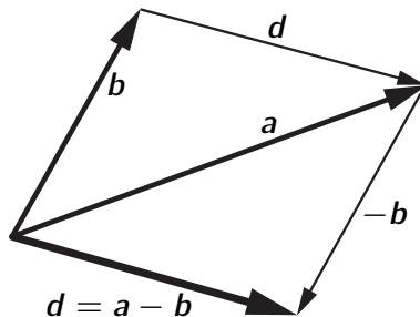
图 11.5: 矢量的减法
