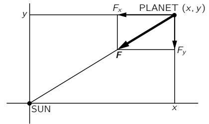
图 9.5: 作用在行星上的太阳引力
